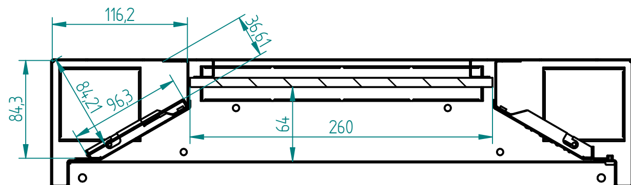
ŘEZ A-A
