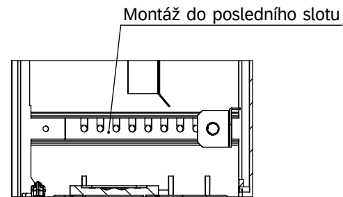
DETAIL D (1 : 5)
