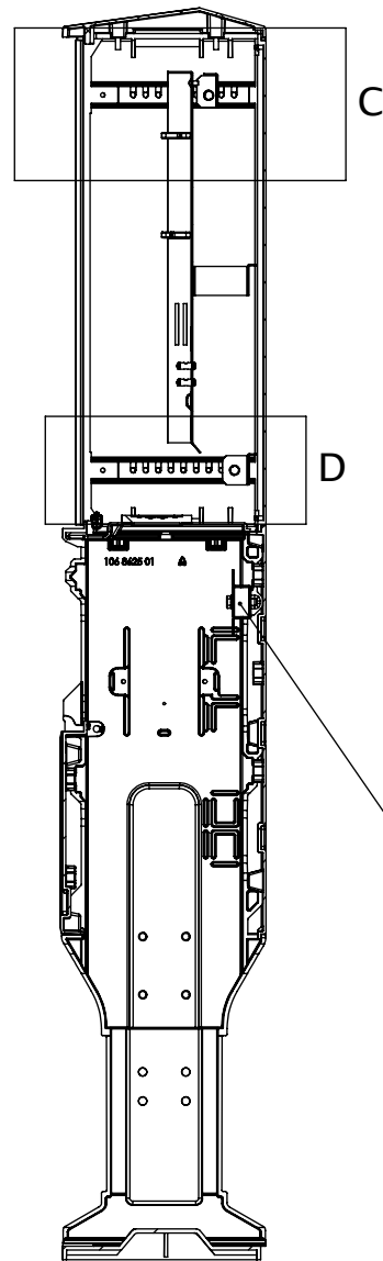
ŘEZ B-B (1 : 10)
