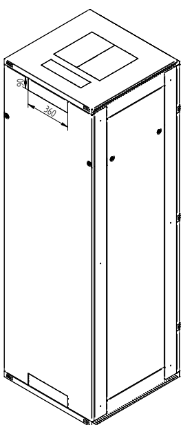
Výkres rozvaděče RMA 54U o půdorysu 800 x 800 mm.
