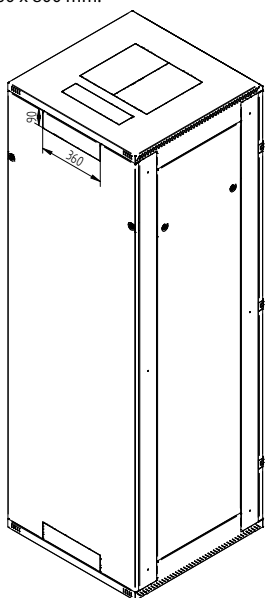
Výkres rozvaděče RMA 52U o půdorysu 800 x 800 mm.
