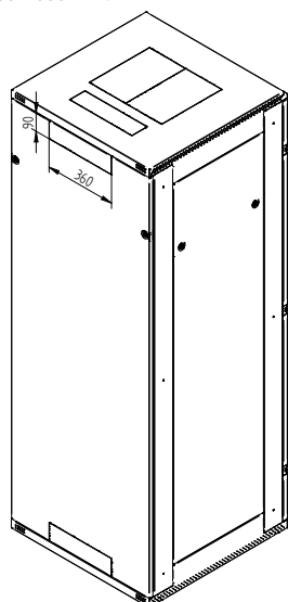
Výkres rozvaděče RMA 47U o půdorysu 800 x 800 mm.
