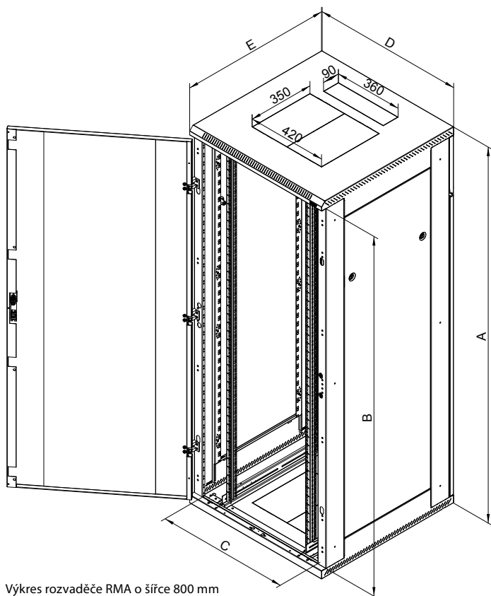
Výkres rozvaděče RMA o šířce 800 mm do výšky rozvaděče 45U včetně.
